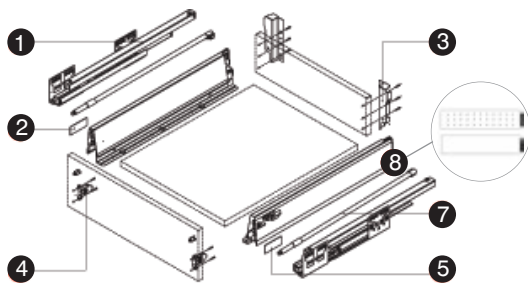
1 Οδηγοί συρταριού (αριστερό/δεξί) 500mm
